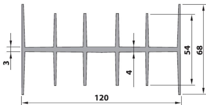
Сечение рядовой секции
